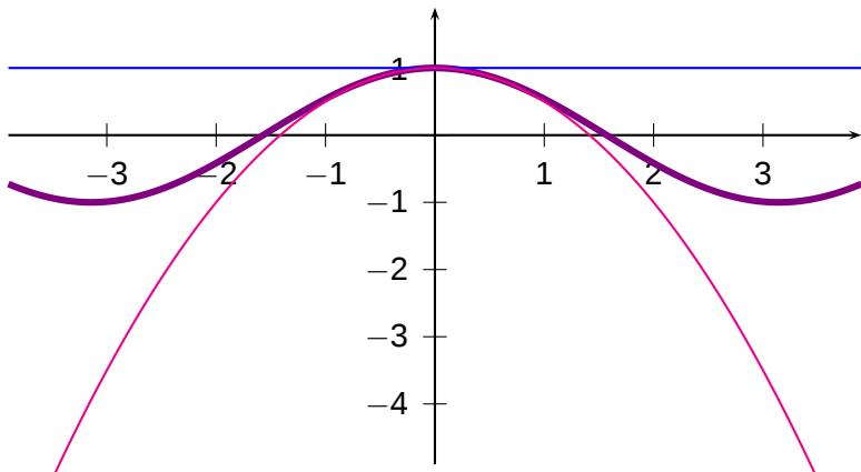
Obrázek: Grafy funkce y = \cos x a jejích aproximací f_1(x) = 1 , f_2(x) = 1 - \frac{x^2}{2} .
