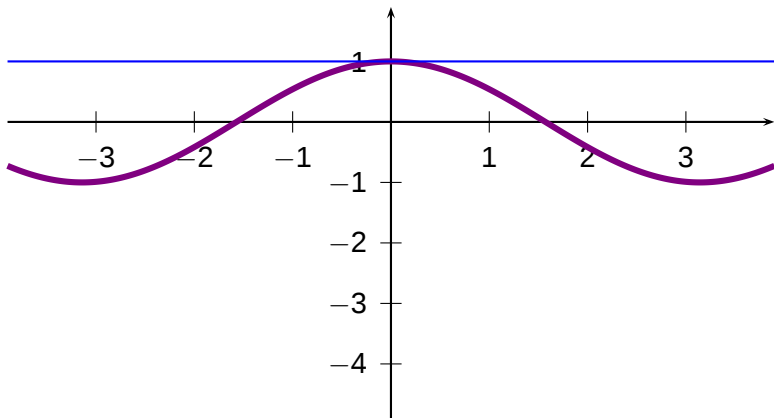
Obrázek: Grafy funkce y = \cos x a její aproximace f_1(x) = 1 .
